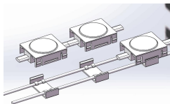
钢丝卡扣
